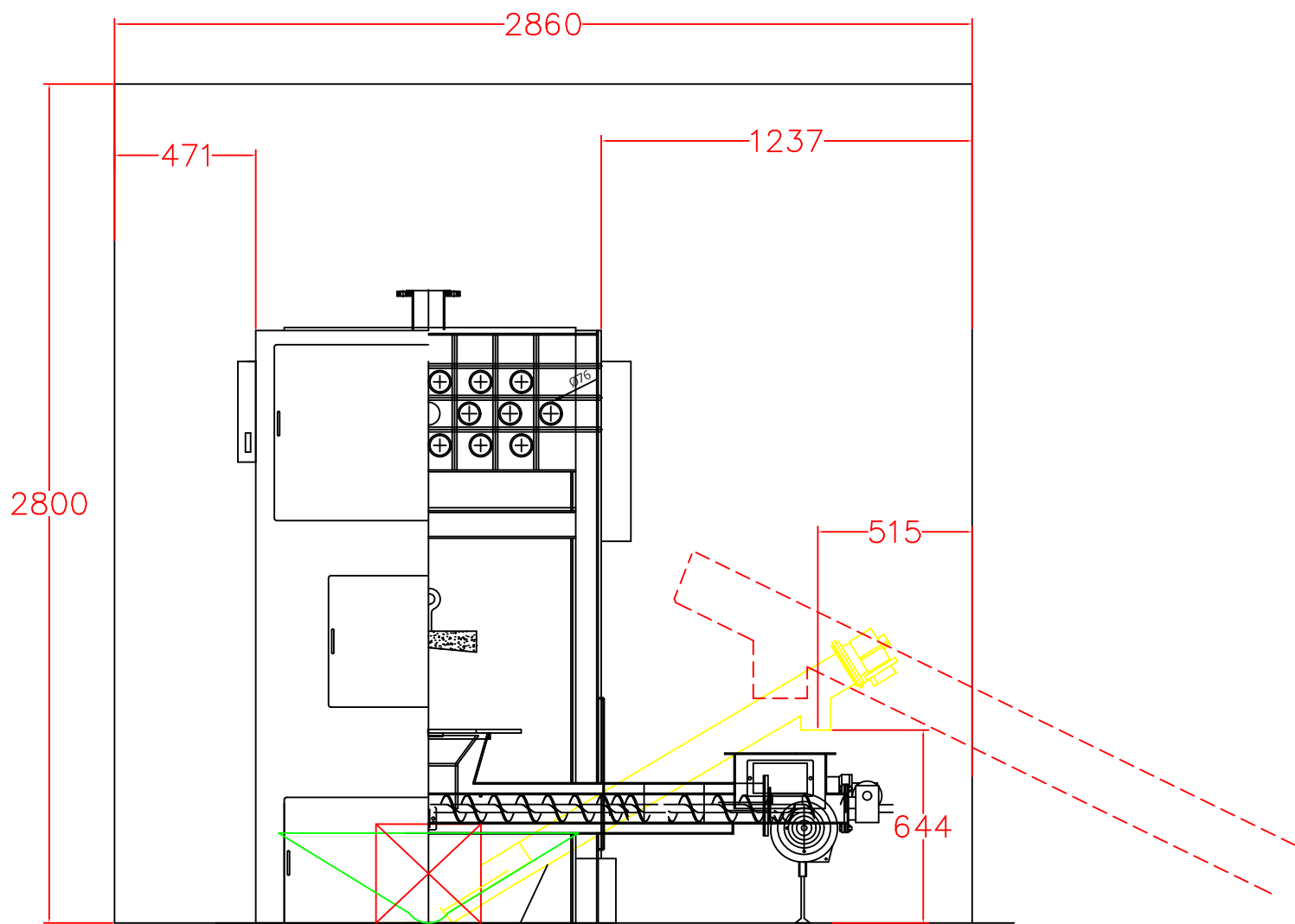
odpopielacz zewnętrzny(skosny)
